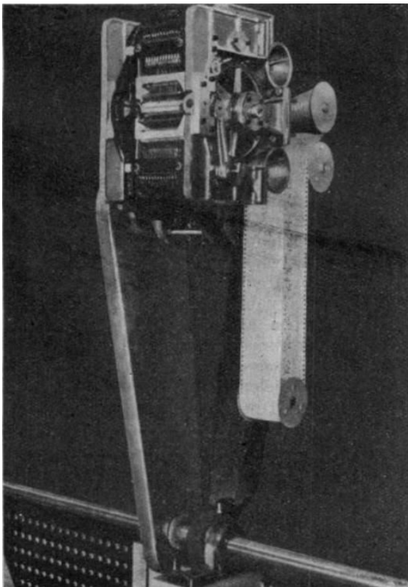
5. ábra. Szalagletapogató berendezés.
