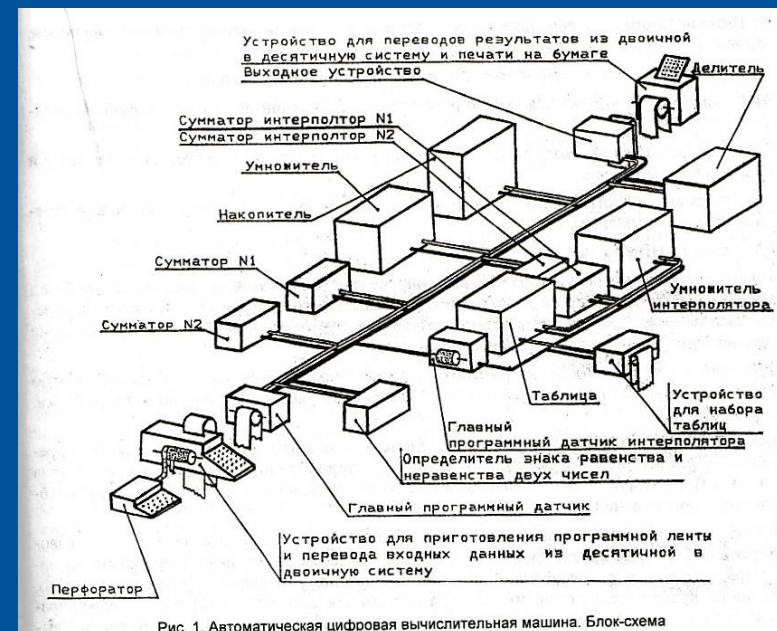
Рис. 1. Автоматическая цифровая вычислительная машина. Блок-схема
